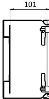
K-K ( 1 : 4 )
