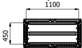
U-U ( 1 : 30 )
